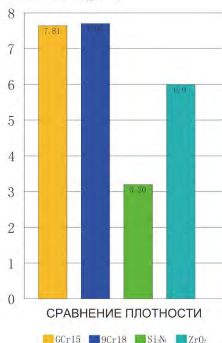
ПЛОТНОСТЬ(g/cm 3 )
