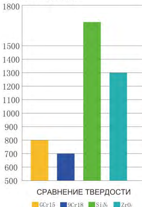
ТВЕРДОСТЬ(HV10)
